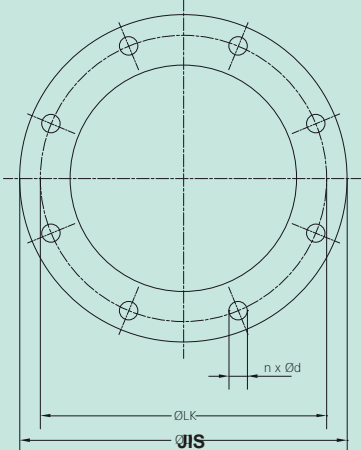
Flange table JIS B
